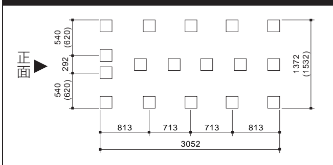
D,WDの基礎図
